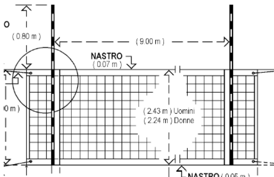
Figura 3 - Sezione
